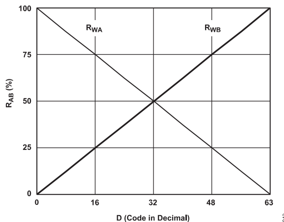
Figure 42. AD5251 R_{WA}(D) and R_{WB}(D) vs. Decimal Code
