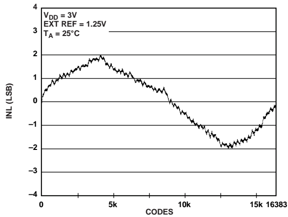
Figure 20. INL AD5648-1
