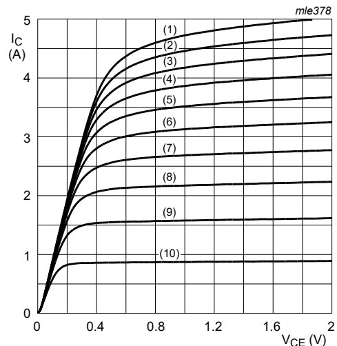
T_{amb} = 25\text{ °C} (1) I_B = 25\text{ mA} (2) I_B = 22.5\text{ mA} (3) I_B = 20\text{ mA} (4) I_B = 17.5\text{ mA} (5) I_B = 15\text{ mA} (6) I_B = 12.5\text{ mA} (7) I_B = 10\text{ mA} (8) I_B = 7.5\text{ mA} (9) I_B = 5\text{ mA} (10) I_B = 2.5\text{ mA}
