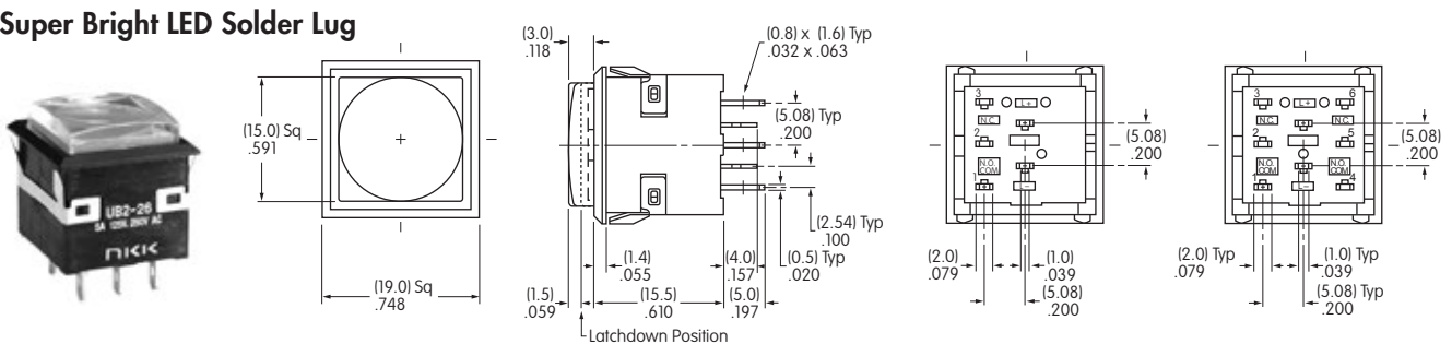
UB226KKW016F-1JF
