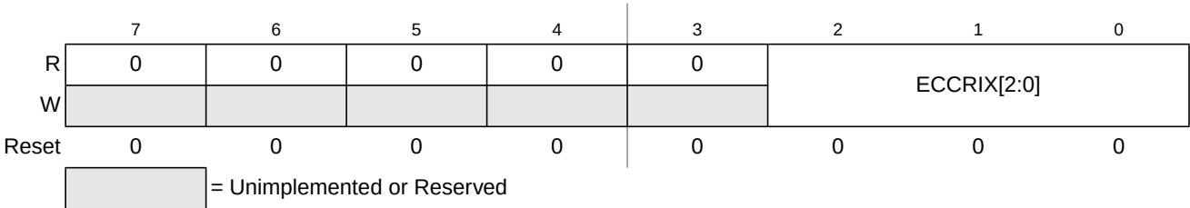
Figure 20-8. FECCR Index Register (FECCRIX)
