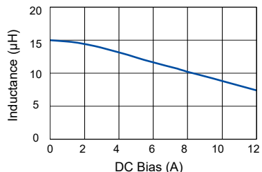
[ ETQP5M100GAK ]
