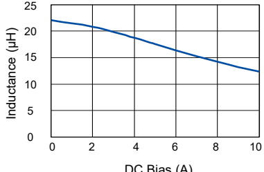
[ ETQP5M101YGK ]
