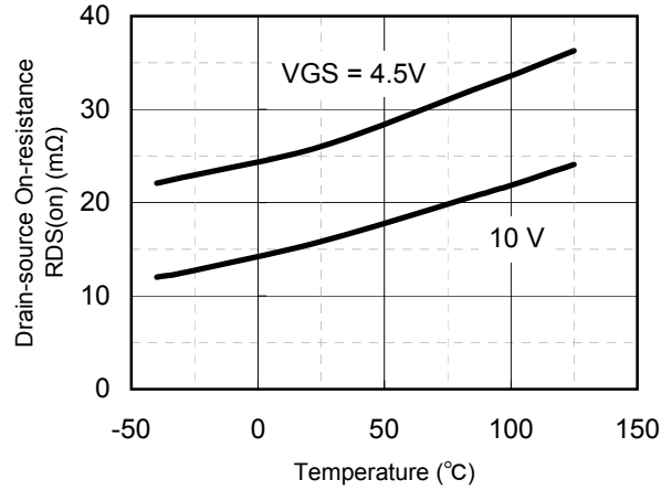
RDS(on) - Ta
