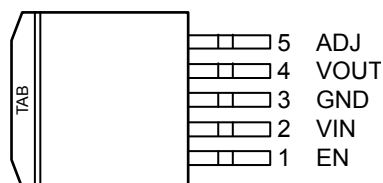
TO-263-5
