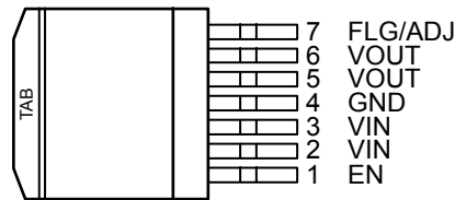
S-PAK-7
