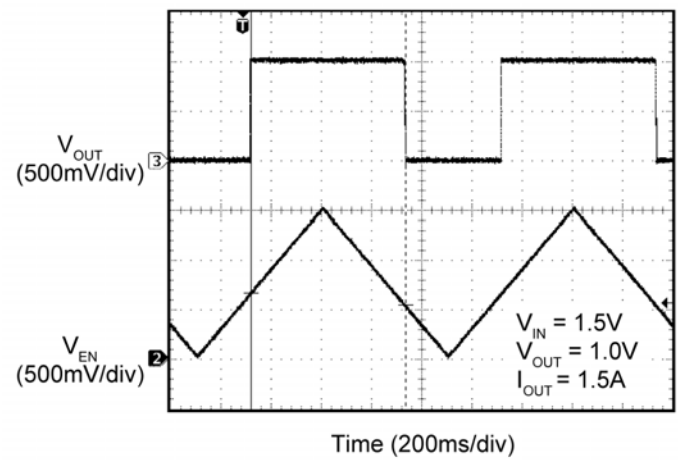
Enable Threshold
