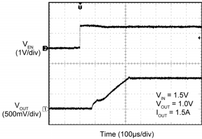
Enable Turn-On
