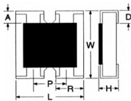
RAVF - 2 Resistors / 4 Terminations (D)
