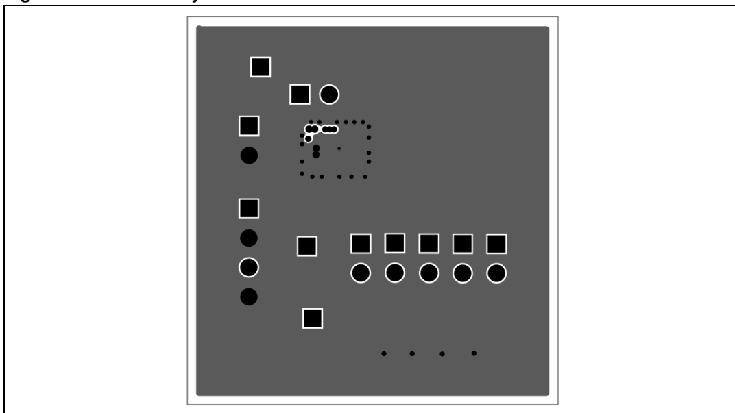
Figure 23. Bottom layer
