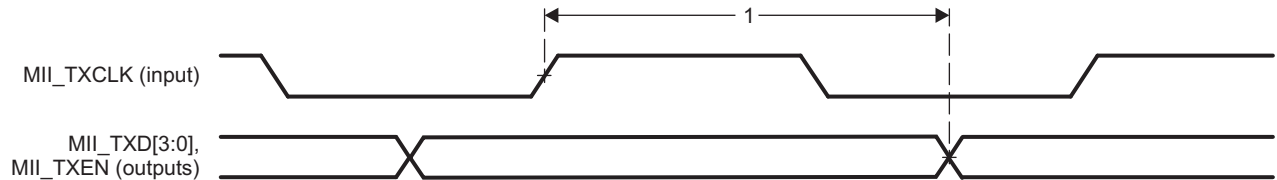
Figure 7-107. PRU-ICSS MII_TXD[3:0], MII_TXEN Timing
