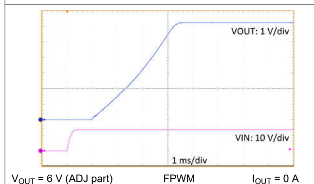
Figure 9-37. Start-up Waveform (EN tied to VIN)
