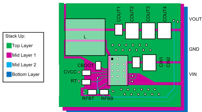
Figure 9-3. LM73605-Q1/6-Q1 Layout Example
