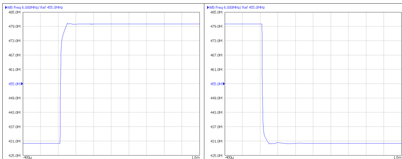
Figure 74. F1 to F2 Switching
