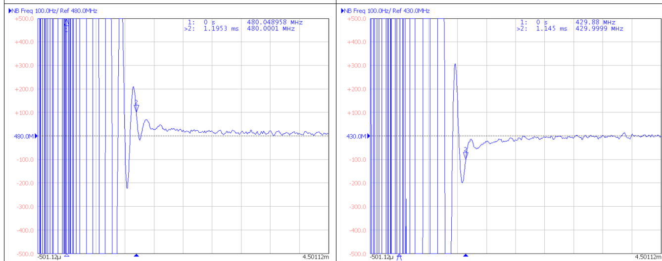
Figure 76. F1 to F2 Switching Time
