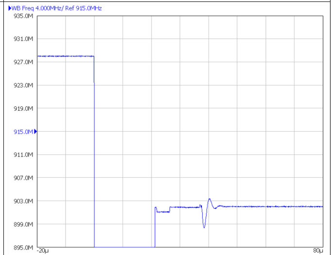
Figure 67. F2 (RX) to F1 (TX) Switching
