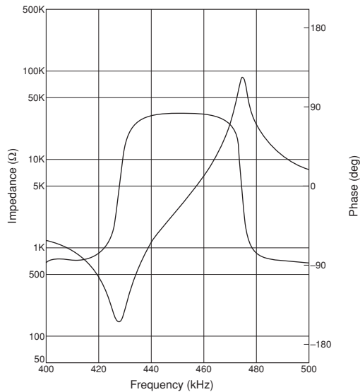
CDBLB455KCAX02-B0
