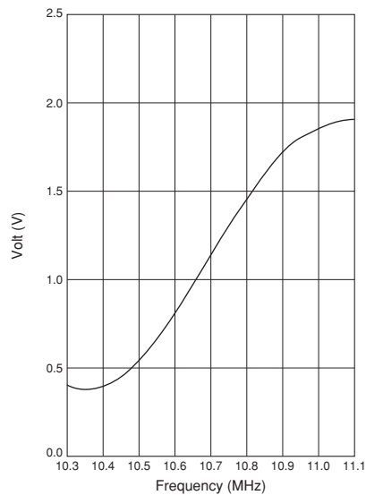
CDSCB10M7GF123-R0
