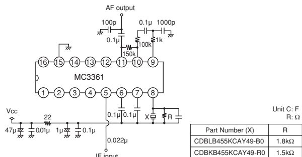
MC3361
