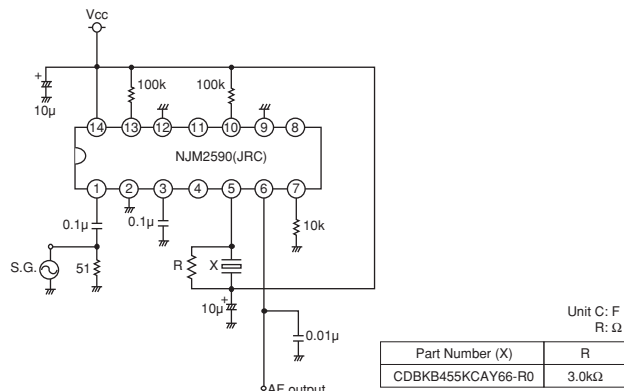
NJM2590
