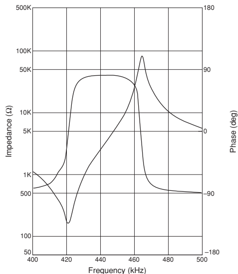
CDBKB455KCAX33-R0
