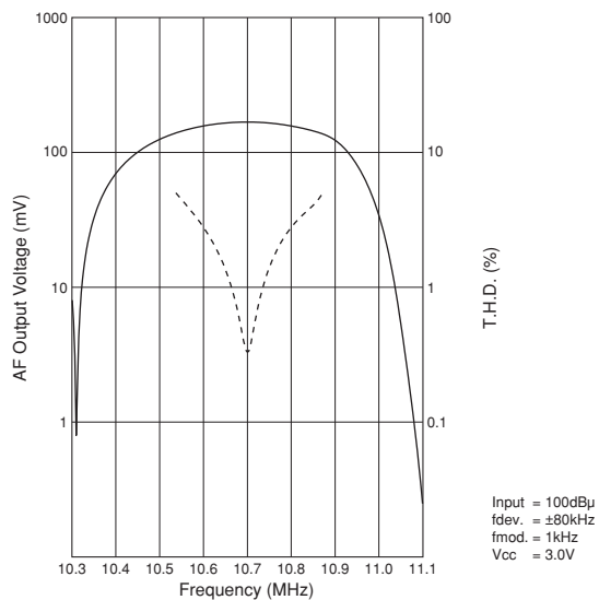
CDSCB10M7GF072-R0
