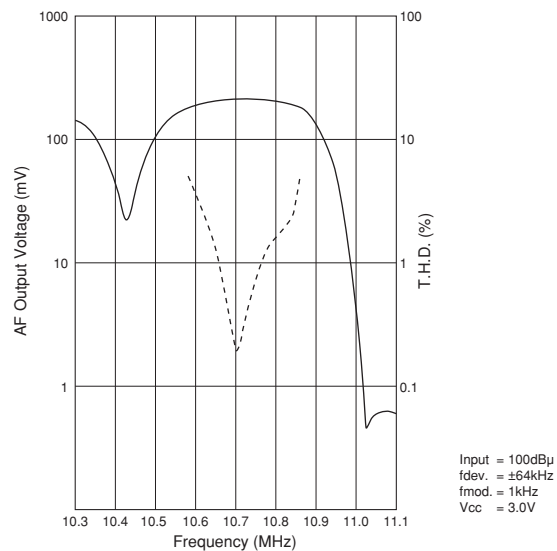
CDSCB10M7GF109-R0
