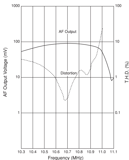
CDSCB10M7GA119-R0
