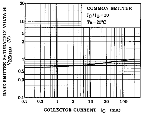
Fig. 8.4 V_{BE(sat)} - I_C
