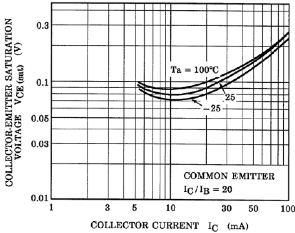
Fig. 10.19 RN1301 V_{CE(sat)}-I_C
