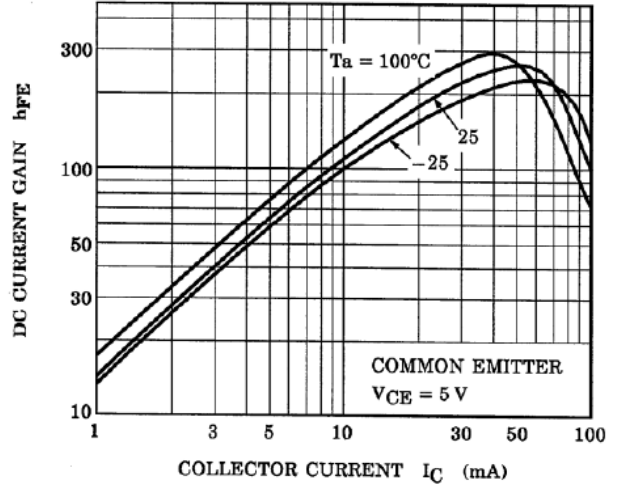
Fig. 10.14 RN1302 h_{FE}-I_C
