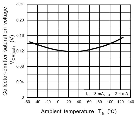
Fig. 11.10 V_{CE(sat)} - T_a
