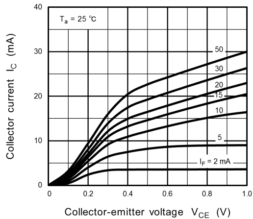
Fig. 11.8 I_C - V_{CE}
