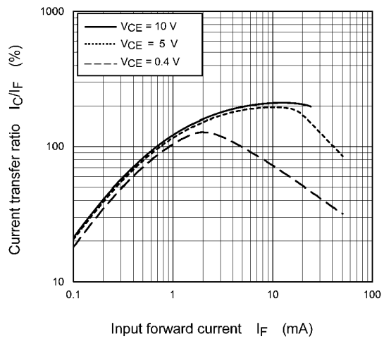
Fig. 11.10 I_C/I_F - I_F
