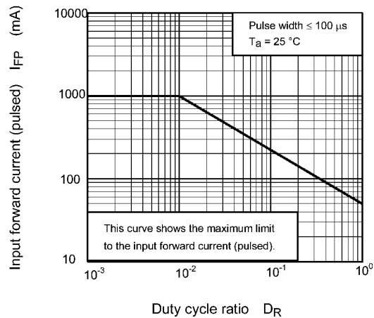
Fig. 11.3 I_{FP} - D_R
