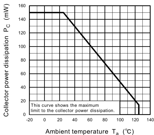
Fig. 11.2 P_C - T_a
