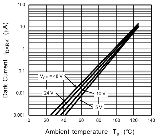
Fig. 12.9 I_{DARK} - T_a
