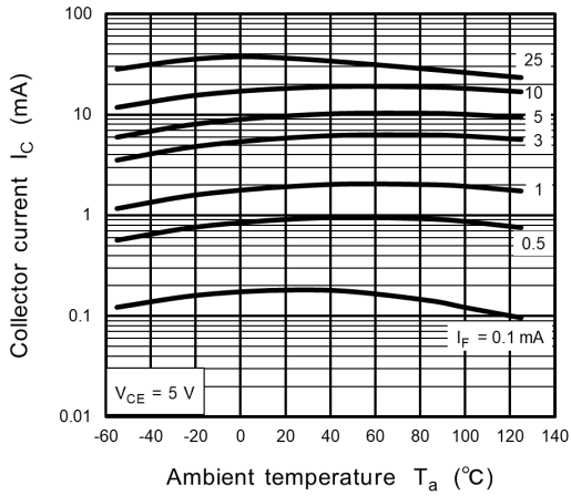
Fig. 12.13 I C - T a
