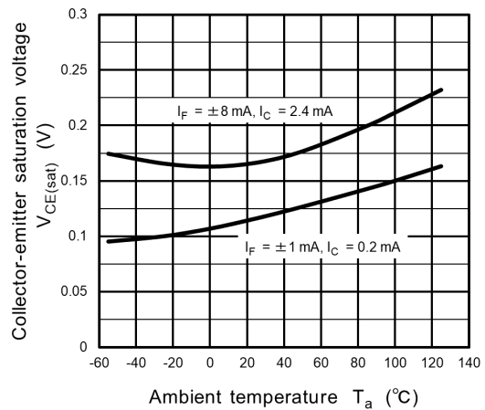
Fig. 12.10 V_{CE(sat)} - T_a
